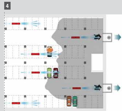
I fumi di incendio vengono estratti The fire smoke is exhausted
