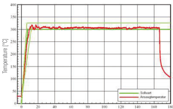
Tempo trascorso da inizio prova Time since beginning of the test
